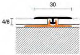
JUNTA SEPARACIÓN Z/4
